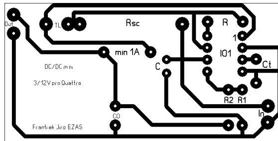
Plošný spoj
