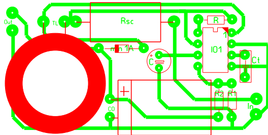
Plošný spoj
