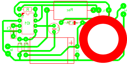
Schéma plošného spoje, strana spojů
